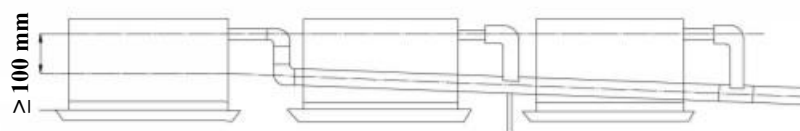
Typ 1 połączenia rur skroplin
