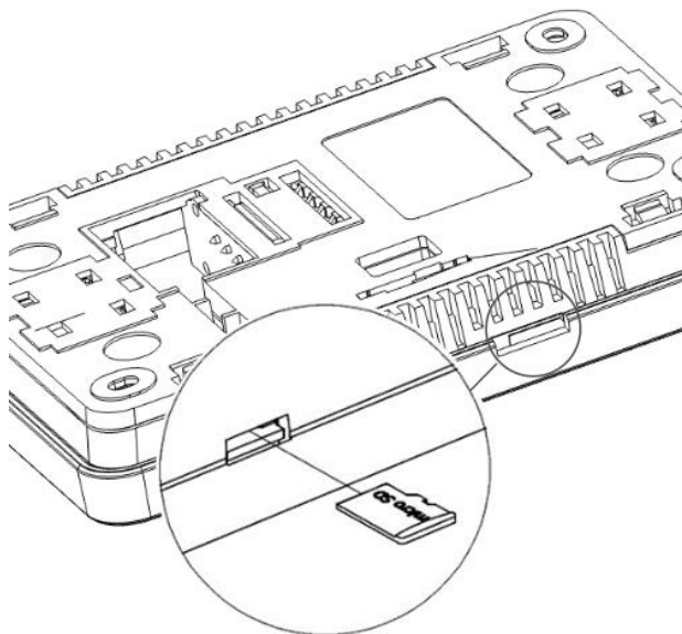
Lokalizacja gniazda pamięci w panelu Black Box.
